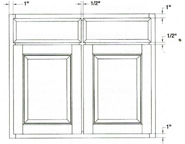
1-3/8" Overlay
