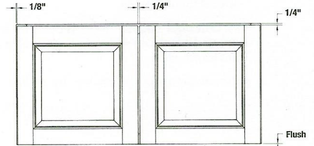
1-3/8" Overlay
